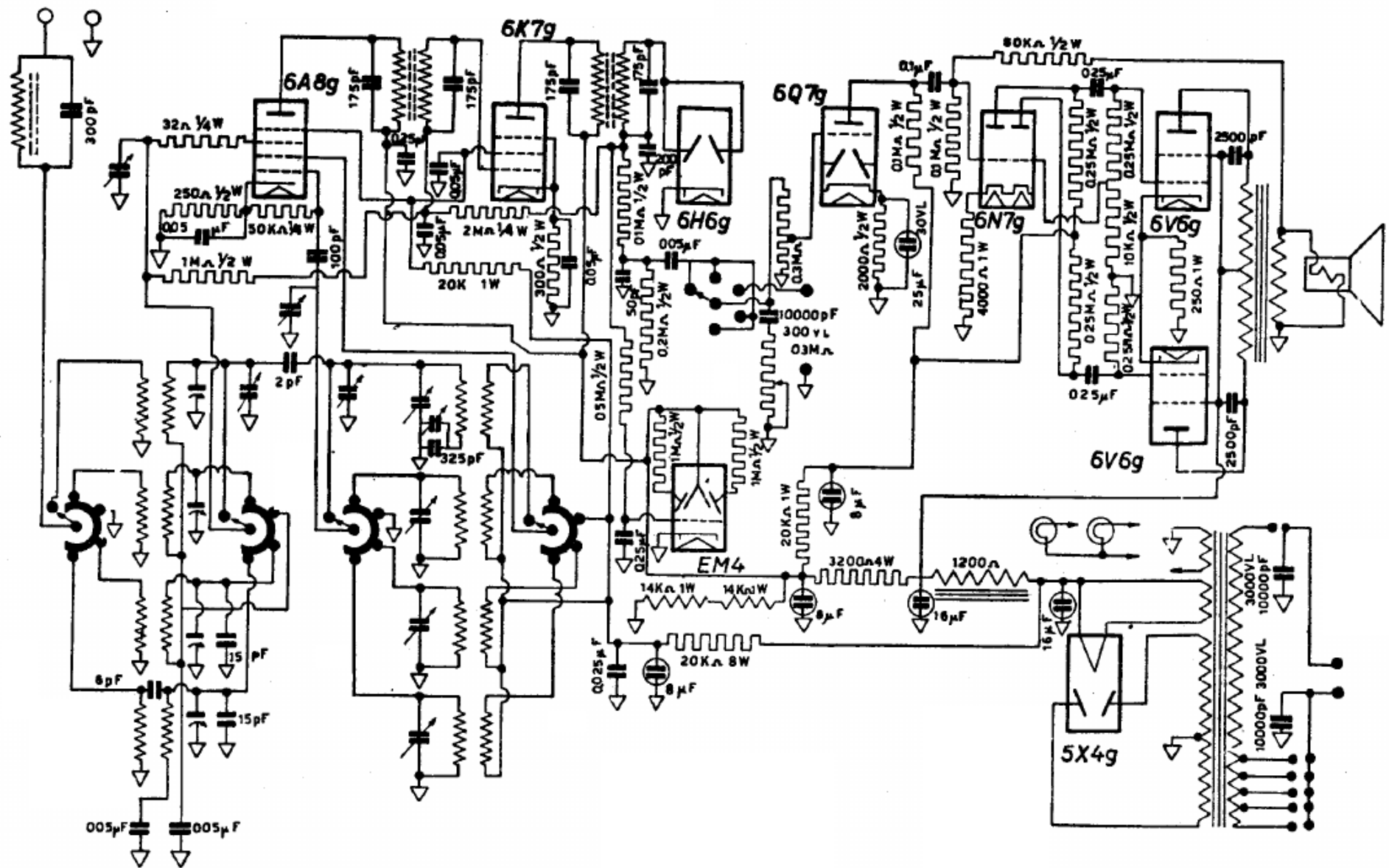
IRRADIO - Mod. DZ 824 - Gamme come modello EX 25. Due 6V6 G finali in controfase, precedute da una 6N7 amplif. BF e invertitrice di fase. Potenza d'uscita circa 12 watt. Ohm eccitazione: 1200. Media frequenza: 450 kc/s. Produzione 1945-46.
